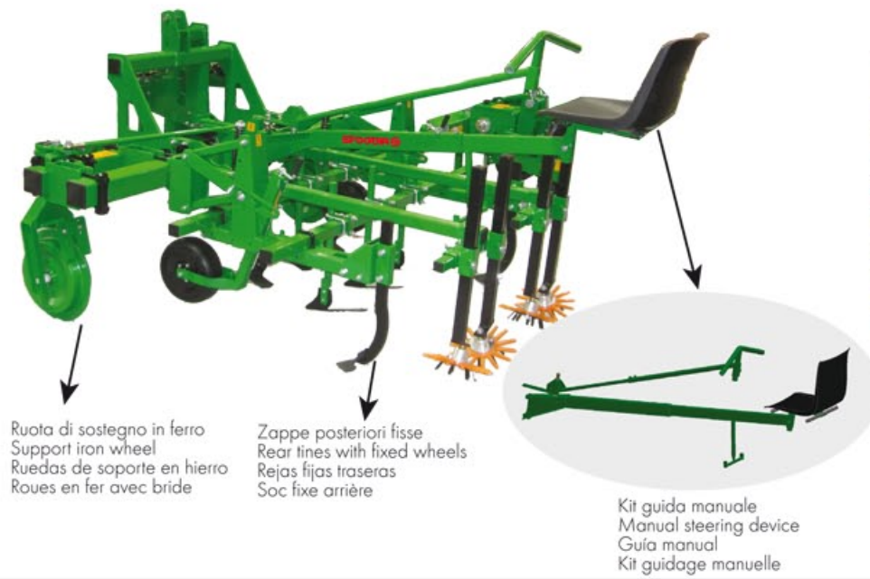
Configurazione per sarchiatura ortaggi Configuration for vegetable cultivation Configuración para el cultivo de las hortalizas Configuration pour la binage de légumes
